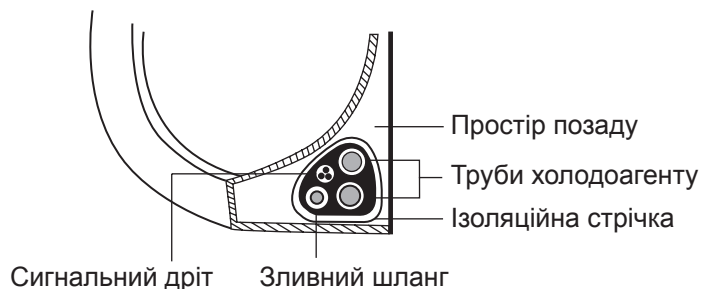
Внутрішній блок
